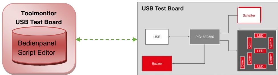
Abbildung 1: Systemarchitektur des USB Test Boards
